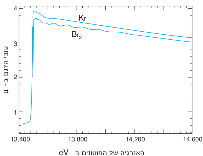
תרשים 6. השוואת אזור סף בליעה של גז מונאטומי (Kr) עם זה של גז מולקולרי ( Br_2 ). על העקומה של הברום מופיעים מאקסימא וומינימא קטנים.
