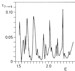
Abb. 3: Quantenmechanischer Versuch: Transmissionswahrscheinlichkeit \tau_{7,9} als Funktion der Einschubenergie E im klassisch-chaotischen Regime.
