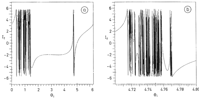
Abb. 2: a) Die Streufunktion I_f in Abhängigkeit vom Winkel \theta_i , den der Dipol zu Beginn mit der x -Achse bildet für E = 1.7, V_0 = 3 und I_i = 2 (vgl. Abb. 1). b) Ein vergrößerter Ausschnitt von a).
