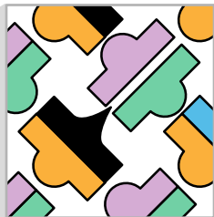
Dopant Site
