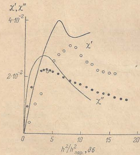
Зависимость вещественной \chi' и мнимой \chi'' частей продольной восприимчивости от мощности накачки для сферы иттриевого граната.
