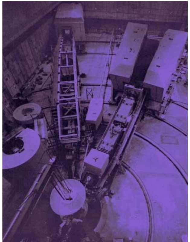
אחת התחנות הסופיות של מאיץ החלקיקים הקווי של סטנפורד (SLAC) שאורכו 3 ק"מ. אלומות מואצות של חלקיקים פוגעים במטרה שבמרכז התחנה ויוצרות מפל של תוצרי חלקיקים. התאוצה הגבוהה מגדילה את המאסה של החלקיקים פי 40,000.
