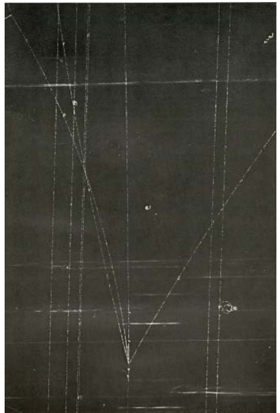
התנגשות גבוהת אנרגיה בין פי-מאזון מהיר לפרוטון ניח (בתחתית התמונה), כפי שהיא מונצחת בתא בוועת, מביאה ליצירת חלקיקים שונים כגון פאיונים, נייטרונים מאזונים ועוד.
