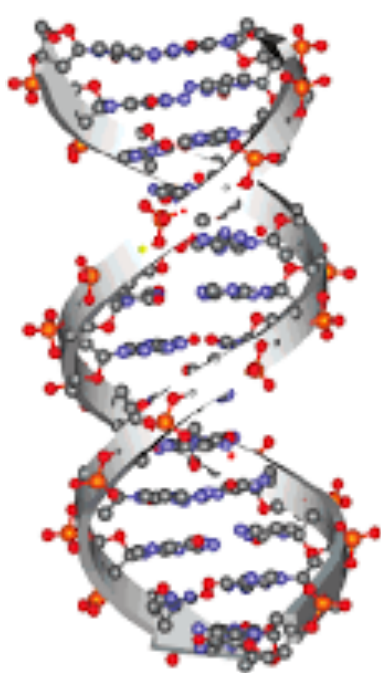
B-DNA
