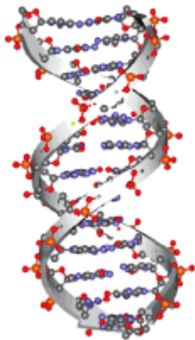
B-DNA
